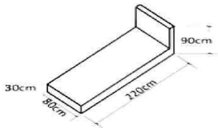
Figura 2.4 Dimensionimi i qivurit për varrin solitar
