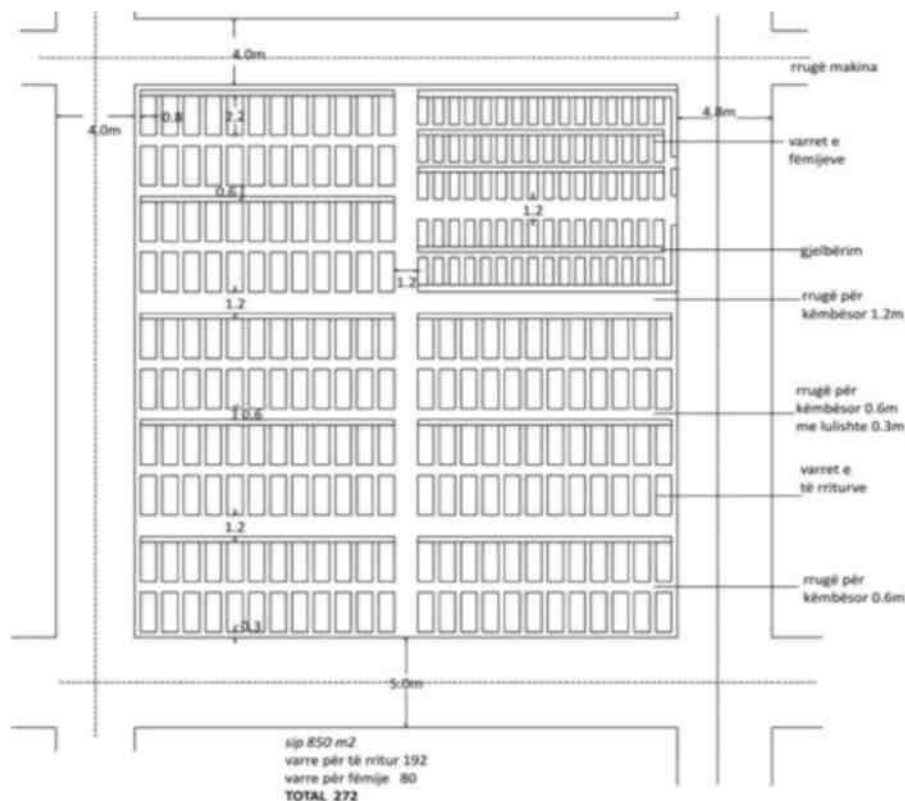
Figura 3.1 Organizimi i një parcele me varre solitare
