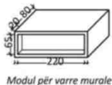
Figura 2.21 Modul gjatësor për varre murale të kufomës
