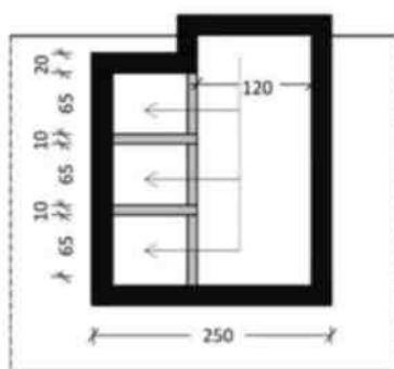
Figura 2.15 T3 –Prerje gjatësore
