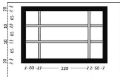
Figura 2.13 T3 –Prerje tërthore
