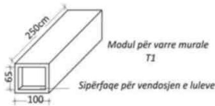
Figura 2.20 Modul tërthor për varre murale të kufomës
