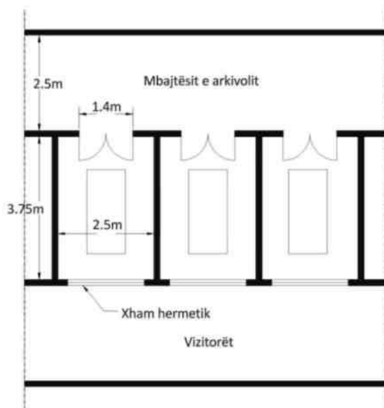
Figura 1.5 Tipologji e projektimit të morgut civil.
