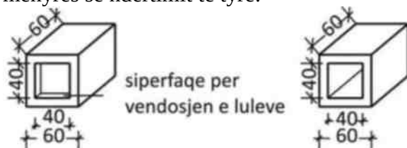
Figura 2.35 Modul i varreve murale të eshtrave
