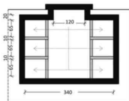
Figura 2.12 T3 –Prerje gjatësore
