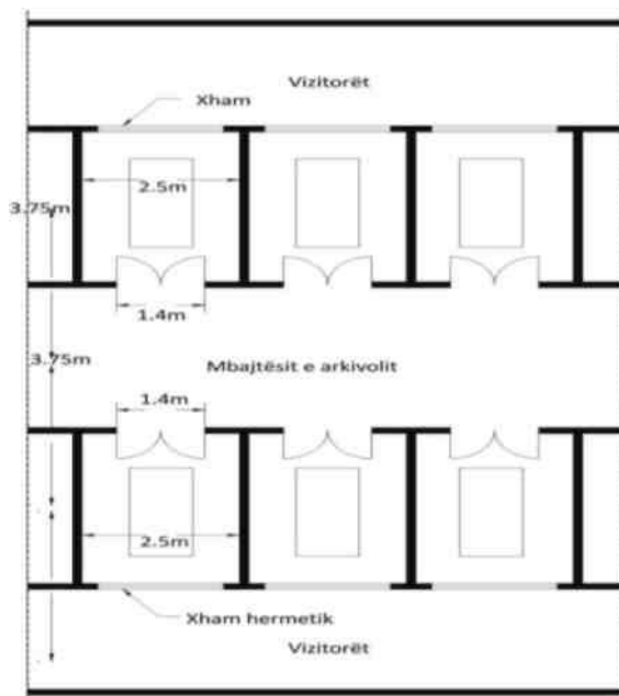
Figura 1.4 Tipologji e projektimit të morgut civil
