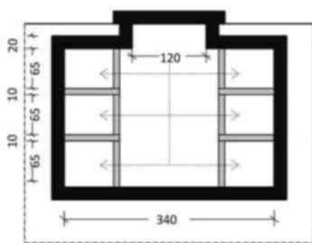
Figura 2.7 T 1 – Prerje tërthore
