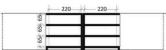
Figura 2.29 T3 – Prerje tërthore
