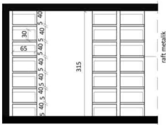
Figura 1.8 Prerje tërthore e magazinës së eshtrave
