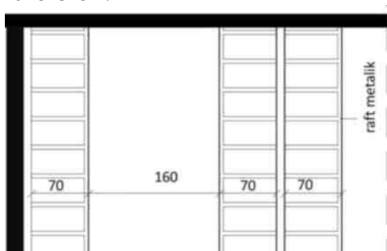
Figura 1.7 Planimetri e magazinës së eshtrave
