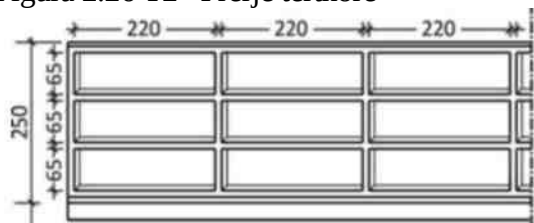
Figura 2.27 T2 – Pamje ballore
