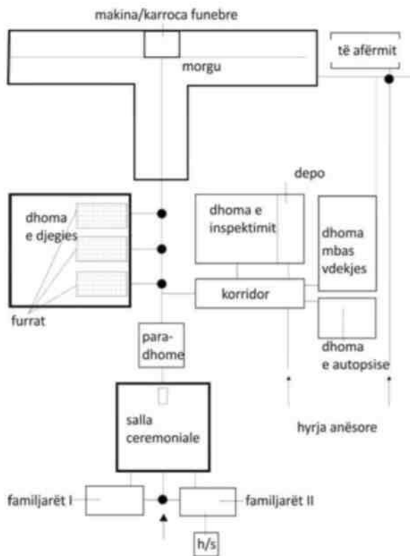
Figura 4.1 Skema e organizimit të krematorit
